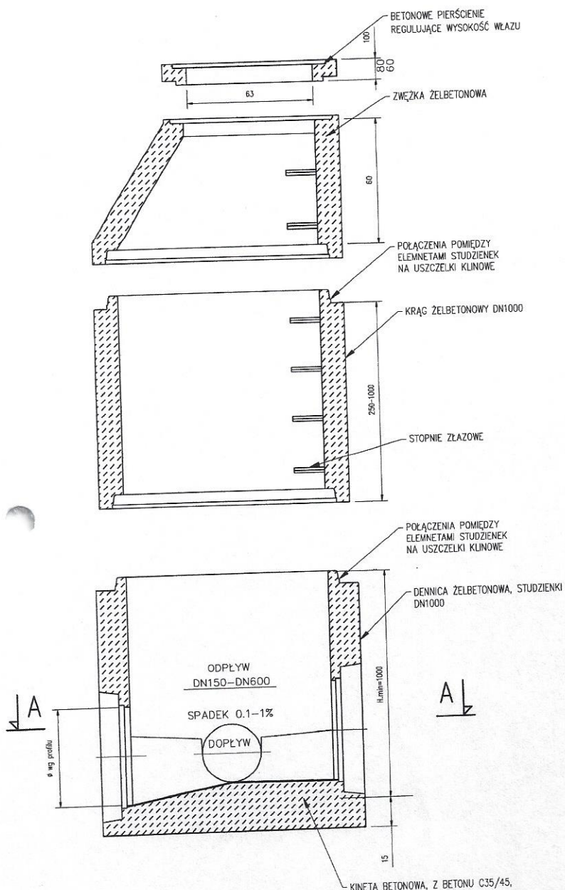
PRZEKRÓJ A-A
