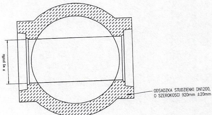
PRZEKRÓJ A-A
