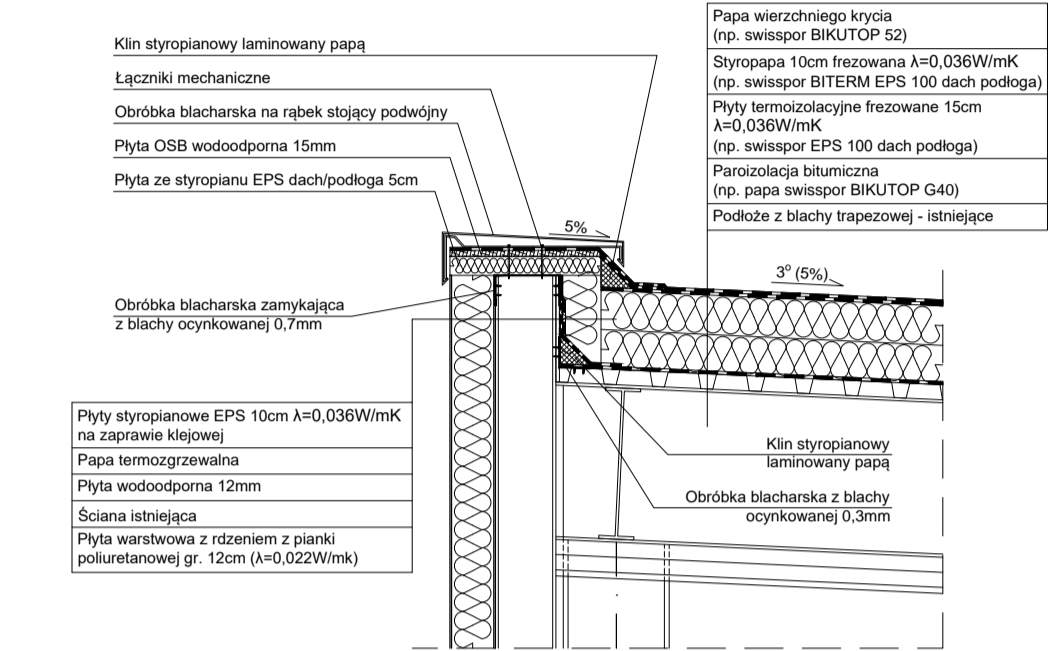
DETAL WYWIETRZAKÓW I PODSTAW DACHOWYCH
