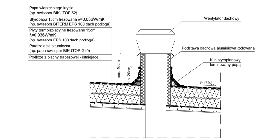
DETAL WYWIETRZAKÓW I PODSTAW DACHOWYCH
