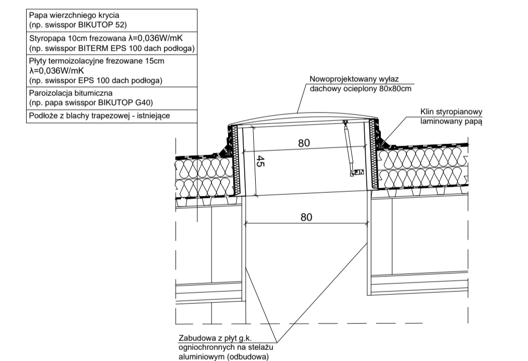
DETAL WYŁAZU DACHOWEGO
